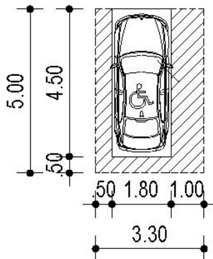
Ελάχιστες διαστάσεις χώρου στάθμευσης ΑΜΕΑ
